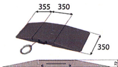
TPS: dimensions en mm.
